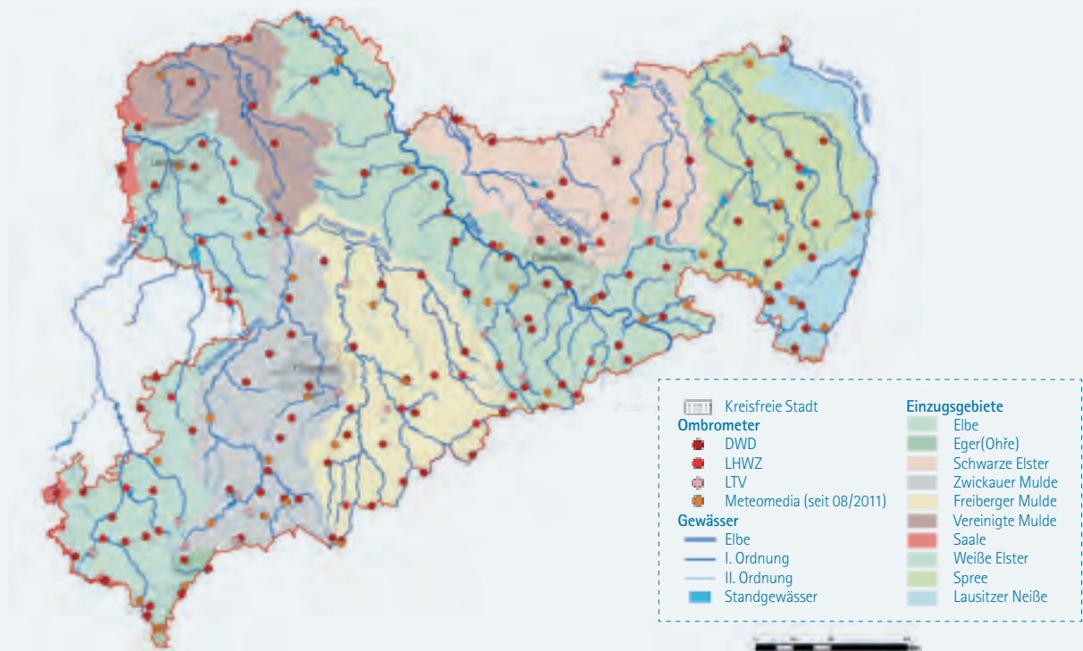
Abbildung 8-3: Ombrometernetz der Flusseinzugsgebiete im Freistaat Sachsen (Quelle: LfULG, Stand 2012)
