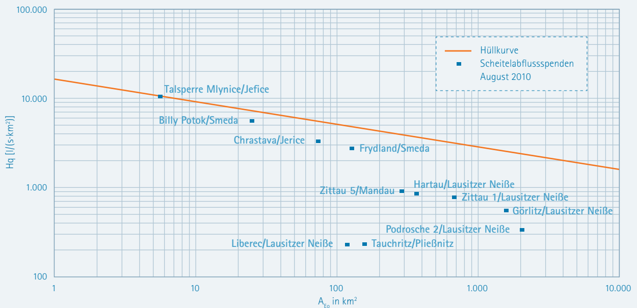
Abbildung 4-13: Scheitelabflussspenden ( H_q ) des Auguthochwassers 2010 für ausgewählte Pegel im Einzugsgebiet der Lausitzer Neiße und aus den Scheitelabflussspenden des Oberlaufs berechnete Hüllkurve
