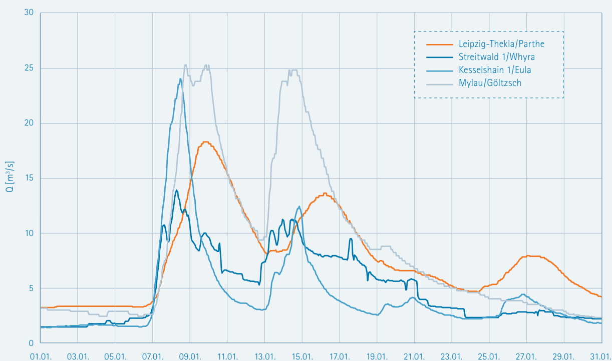
Abbildung 4-64: Abflussganglinien für Januar 2011 an den Pegeln der Pleißenbäche Parthe, Whyra mit Eula sowie dem Weiße-Elster-Nebenfluss und Göltzsch für den Zeitraum 01.01.–31.01.2011
